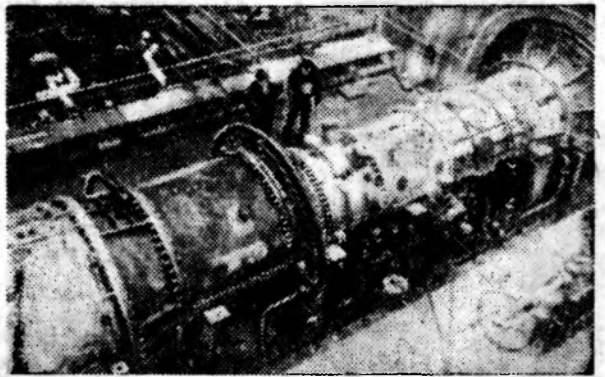
В Ленинграде в объединении «Невский завод имени В. И. Ленина» досрочно изготовлен первый серийный газоперекачивающий агрегат мощностью 25 тысяч киловатт. Перенец новой серии, предназначенный для экспортной магистрали Уренгой — Помары — Ужгород, прошел испытания на стенде предприятия.
