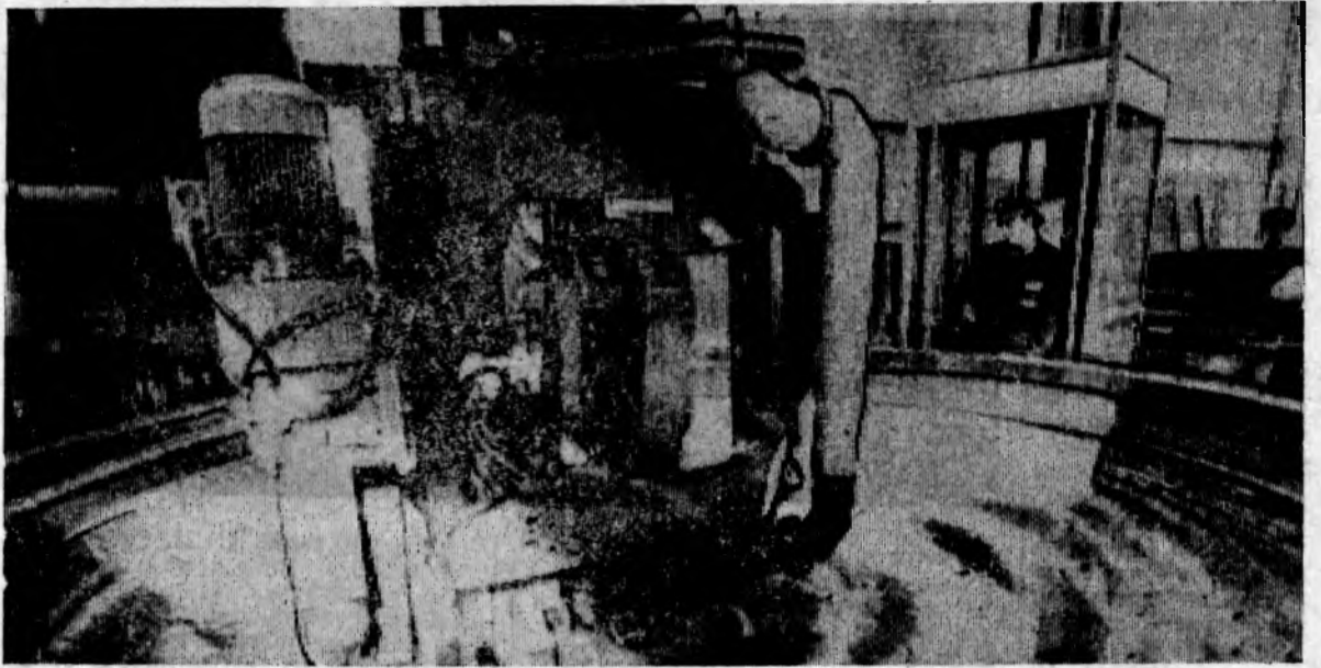
На снимке: шлифовка внутренней поверхности днища корпуса реактора. Эта работа выполняется недавно пущенным на «Атоммаше» уникальным станком. Фото А. Бурдюгова.
