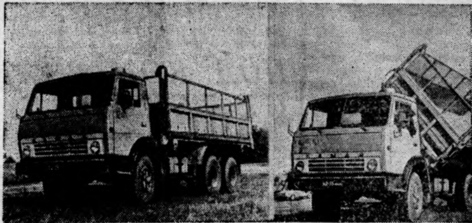
Два самосвала марки «КамАЗ-55102» собраны в экспериментальном цехе Минского автомобильного завода. Это уже второй образец машин сельскохозяйственного назначения, разработанный для КамАЗа конструкторами Московского имени Лихачева и Минского автозаводов. У нового автомобиля шасси — зловское, платформа и самосвальная установка — мазовские. Трехосный «КамАЗ-55102» имеет два ведущих моста. Самосвальная установка позволяет осуществлять ускоренную разгрузку на любую из трех сторон. Грузоподъемность автосамосвала с прицепом составляет 15 тонн.
