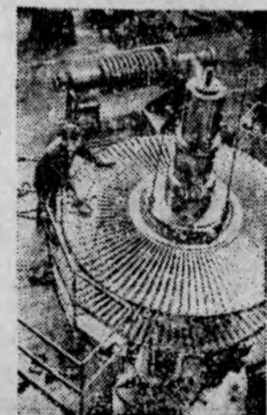
Ленинград. Металлический завод имени XXII съезда КПСС — крупнейший поставщик энергетического оборудования. Агрегаты, созданные на этом предприятии, работают на многих электростанциях Советского Союза, в странах Европы, Азии и Африки. На снимке: слесарь-сборщик В. А. Гринев производит насадку дисков ротора паровой турбины. Фото П. Федотова. (Фотохроника ТАСС).
