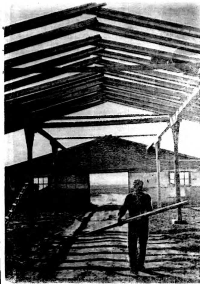
В этом году в колхозе «Искра» вступит в строй еще один механизированный коровник (на снимке). В нем разместятся 400 животных. Работу ведет бригада Цимлянского СМУ «Межколхозстрой», которую возглавляет К. П. Богрецов. Сейчас строители устанавливают перекрытия. А весь объект они намерены сдать в июле.
