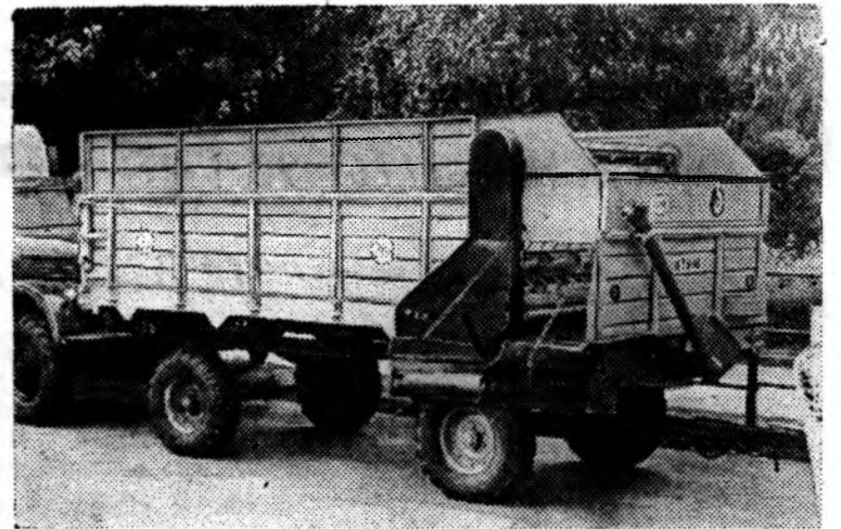
МОСКВА. Этот новый универсальный кормораздатчик «КТУ-10», который сейчас демонстрируется на Выставке достижений народного хозяйства СССР, — более совершенная машина, чем ее предшественники. С ее помощью можно накормить до 800 коров. Конструкция кузова машины, вмещающего 5,5 кубометра корма, позволяет сгружать корм в любую сторону.
