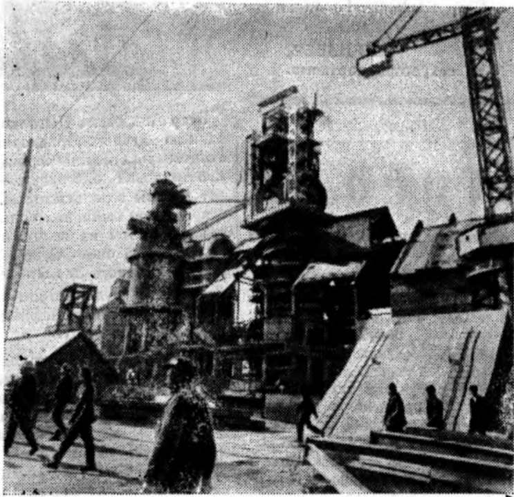
ИРАН. Строительство металлургического завода в Исфагане, сооружаемого при техническом содействии Советского Союза, идет полным ходом. На строительной площадке поднялись конструкции доменной печи, монтируются важнейшие узлы предприятия.
