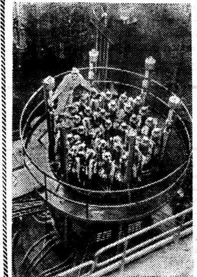
Реактор Нововоронежской атомной электростанции.
