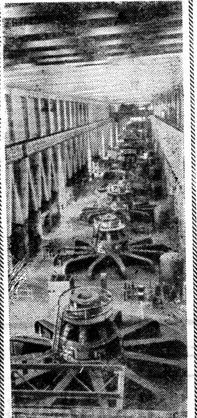
Братская ГЭС. Машинный зал.
