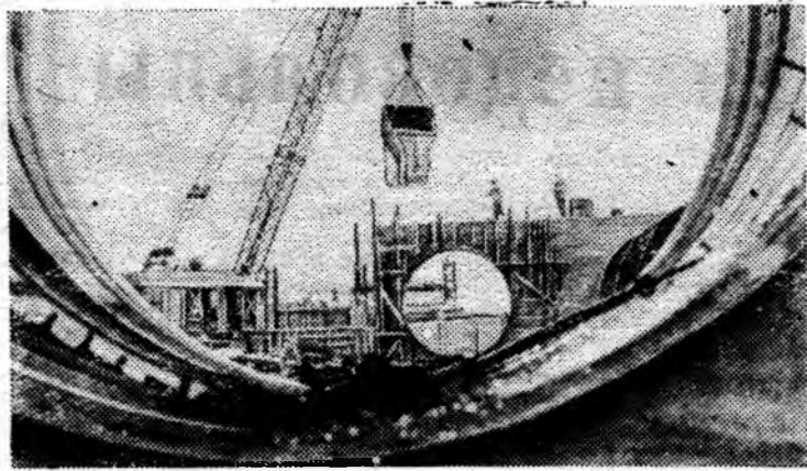
Ирригаторы Ставрополя сооружают Кубань-Калаусскую оросительную систему. С вводом в строй только первой ее очереди тридцать пять тысяч гектаров плодородной земли засухливой зоны получат воду. На гидроузле будет возведено несколько электростанций.
